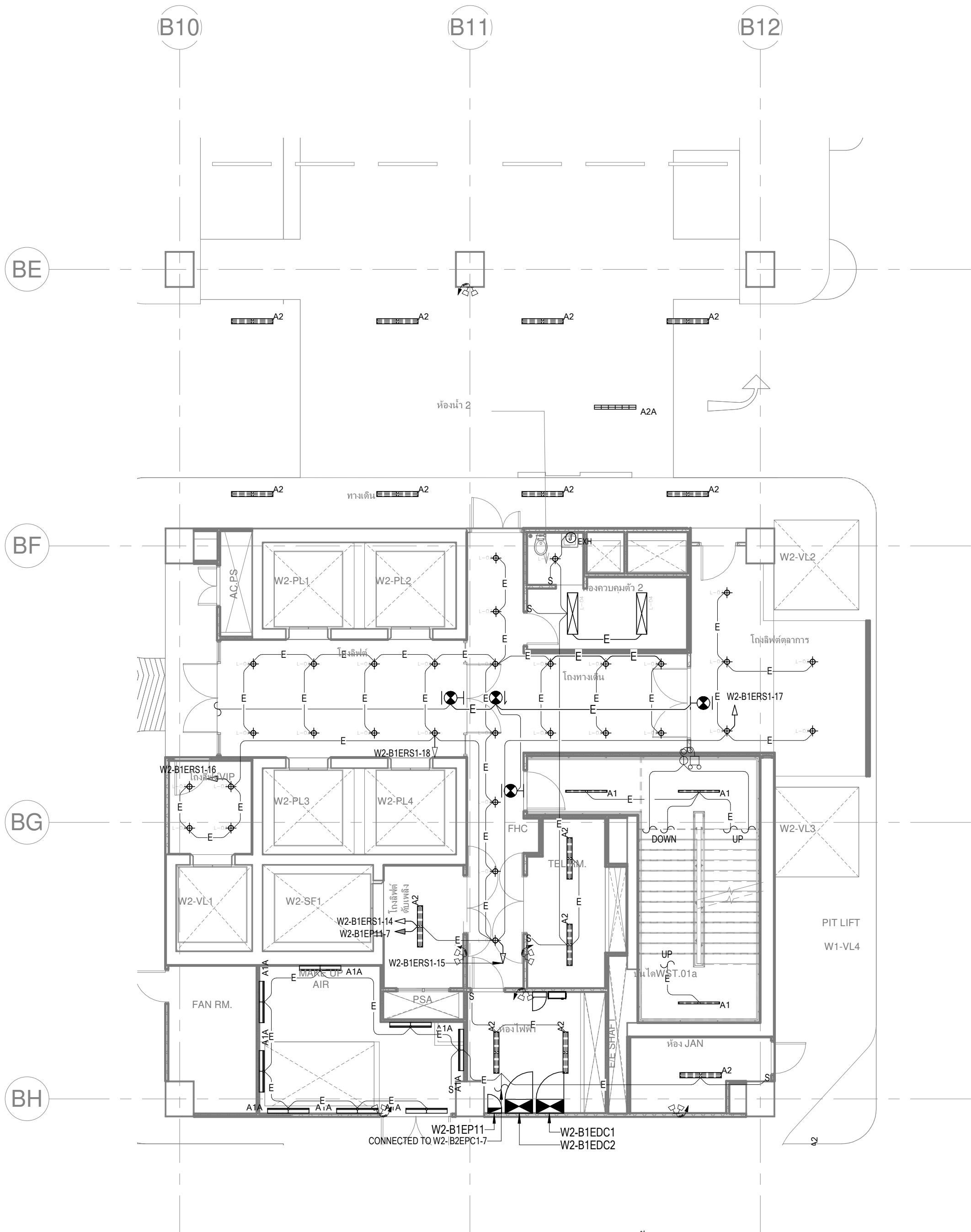
แบบขยายระบบไฟฟ้าแสงสว่าง บริเวณ Core W2 สำหรับชั้นใต้ดิน 1 มาตราส่วน 1:100
