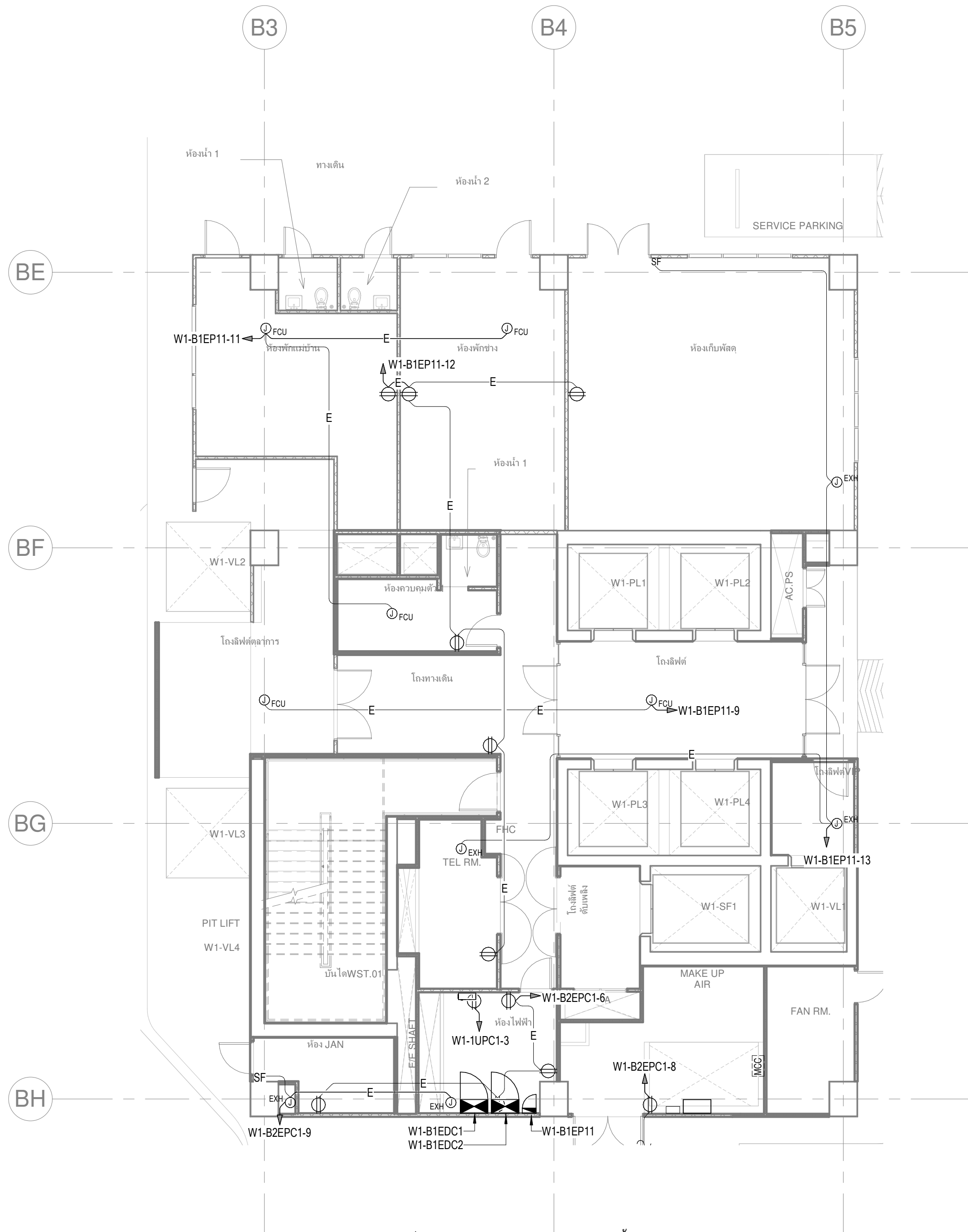
แบบขยายเต้ารับไฟฟ้า บริเวณ Core W1 สำหรับชั้นใต้ดิน 1 มาตราส่วน 1:100
