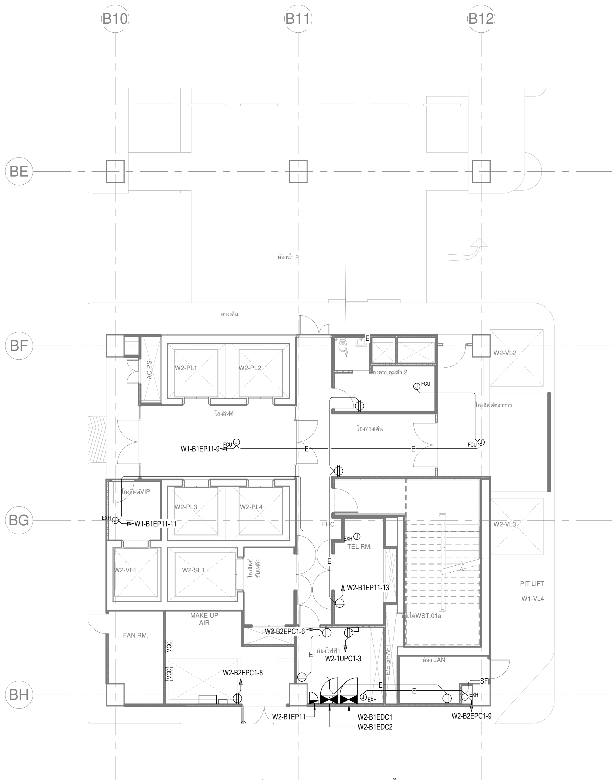
แบบขยายเต้ารับไฟฟ้า บริเวณ Core W2 สำหรับชั้นใต้ดิน 1 มาตราส่วน 1:100
